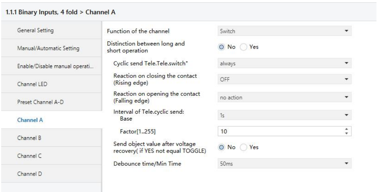
图 5.7 “Switch”参数设置界面（不区分长/短操作）
