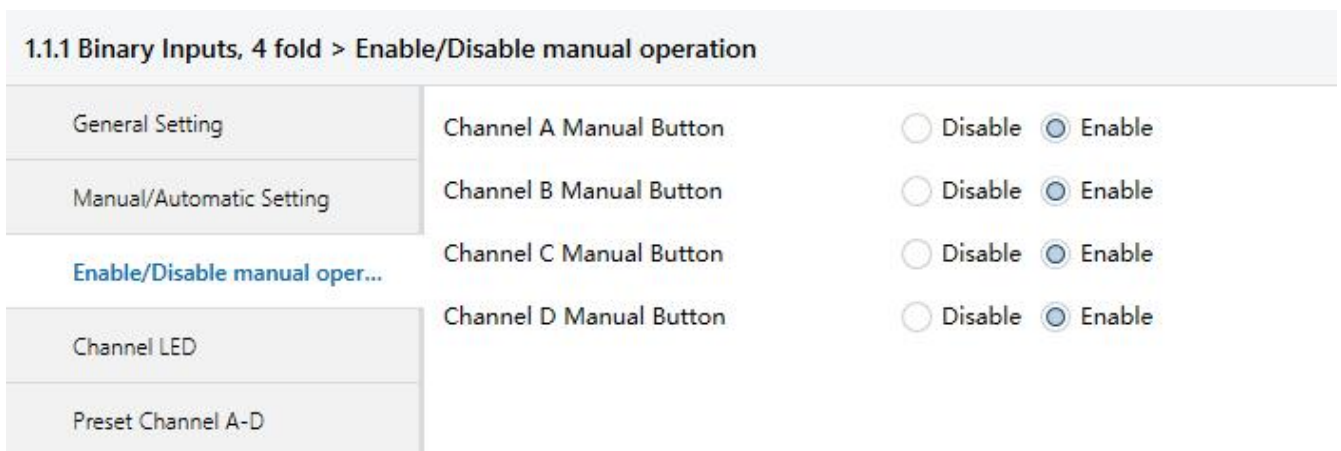
图 5.3 “Enable/Disable manual operation”参数设置界面
