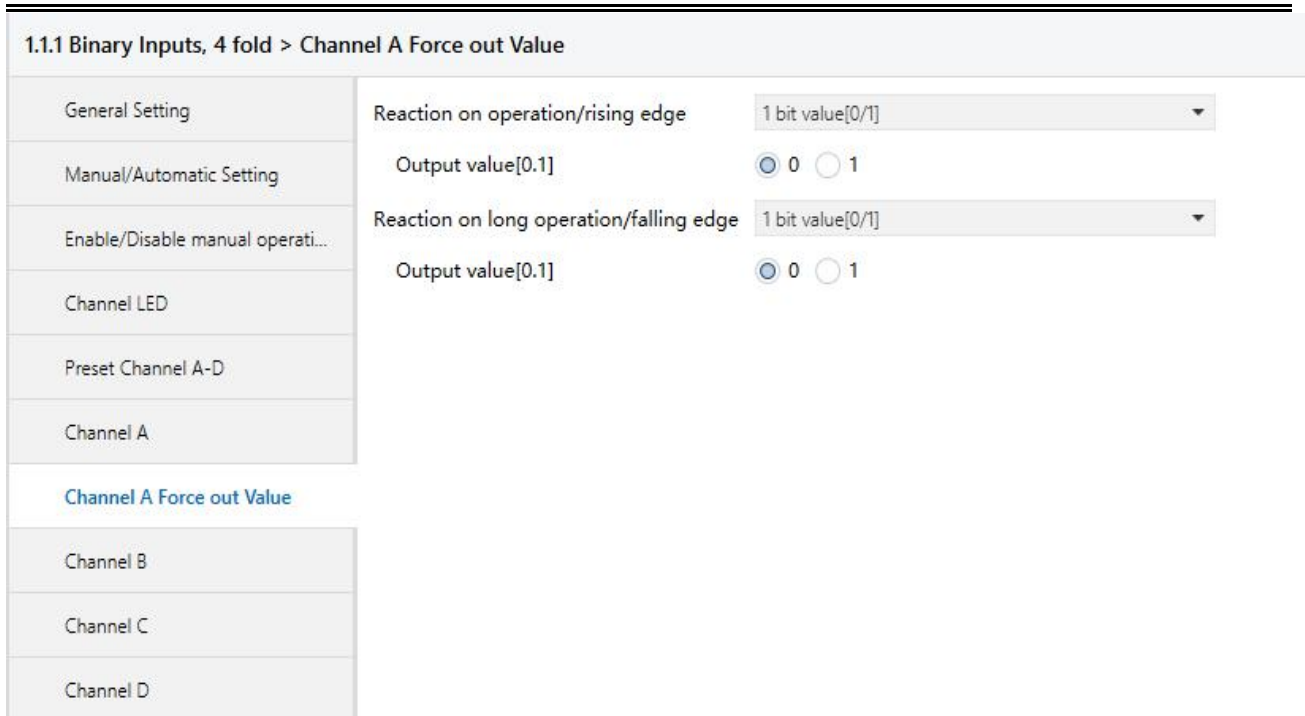
图 5.11 (3) “Force out Value, X”参数设置界面
