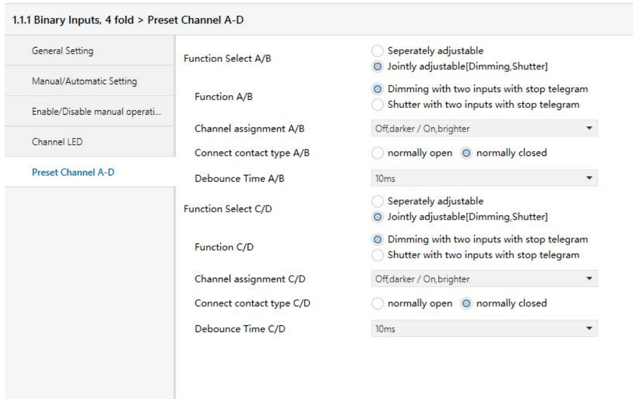
图 5.5 (2) “Preset Channel A~D”参数设置界面（组合工作方式）
