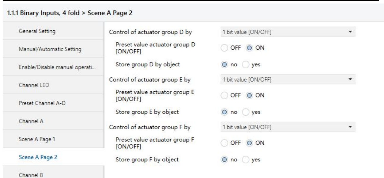
图 5.12 (2) “Scene X Page 1/2, X”参数设置界面
