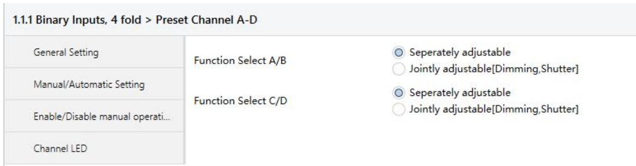
图 5.5 (1) “Preset Channel A~D”参数设置界面（独立工作方式）
