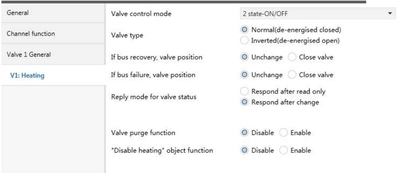
Fig. 4.29 Parameter window "Vx: Heating"
