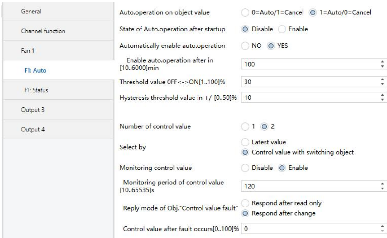
Fig. 4.21 Parameter window "F1: Auto."
