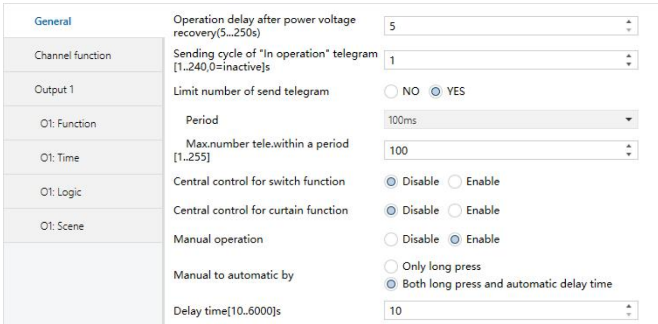
Fig. 4.1 Parameter window “General”
