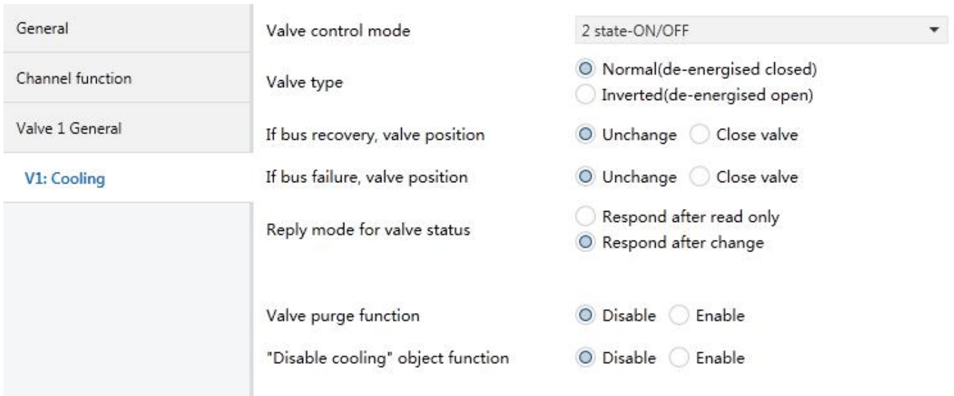
Fig. 4.30 Parameter window "Vx: Cooling"
