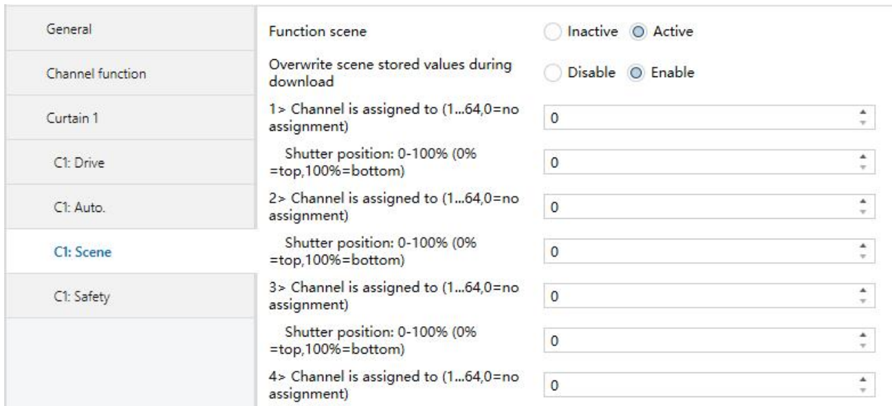
Fig. 4.17 Parameter window “Cx: Scene”
