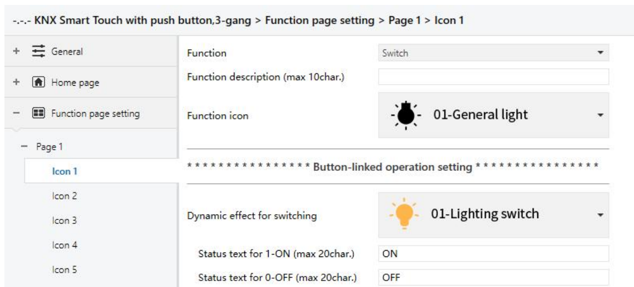
Fig.5.6.2.1 (1) Parameter setting of switch function
