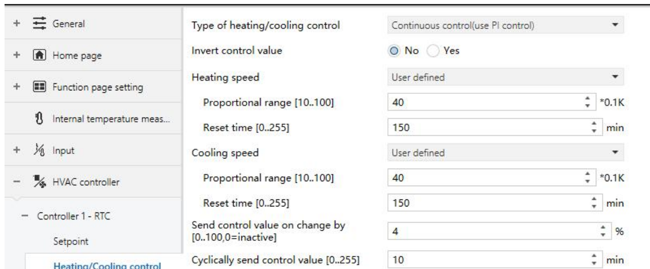
Parameter setting of “Continuous control(use PI control)” Fig.5.4.1.2 “Heating/Cooling control” parameter window
