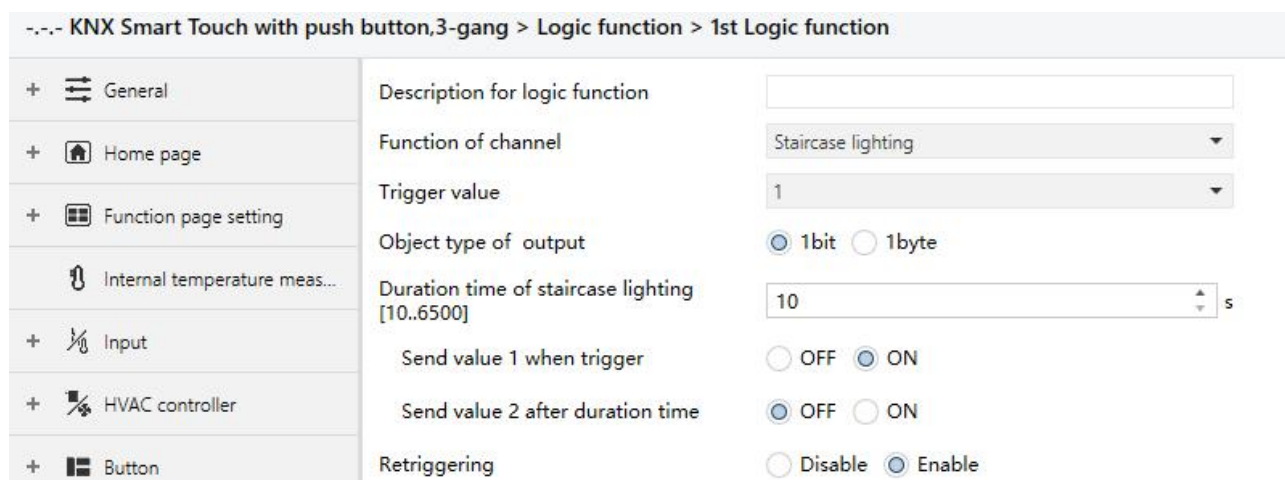
Fig.5.8.7 “Staircase lighting” parameter window
