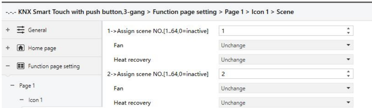
Fig.5.6.2.4(2) Ventilation system-scene parameter window
