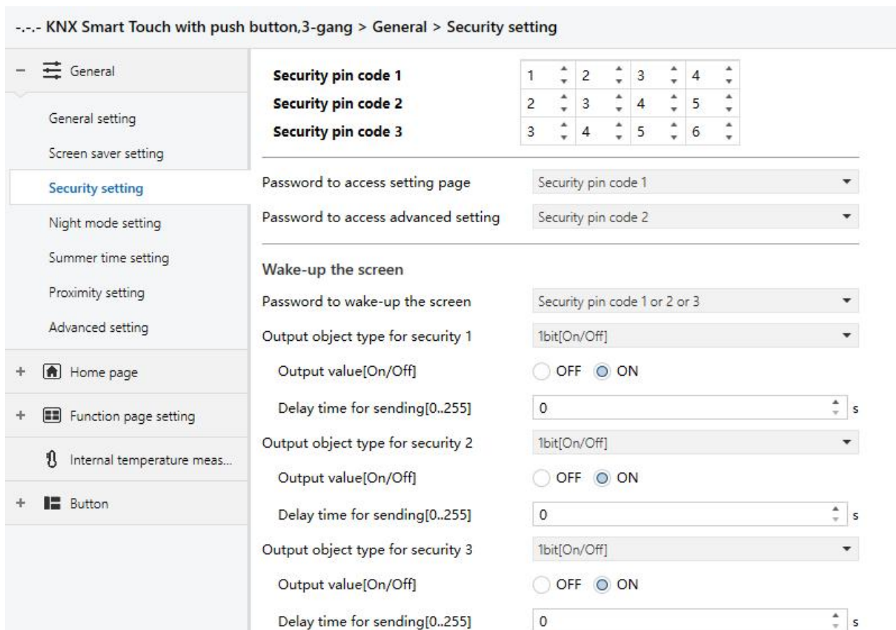
Fig.5.1.3 “Security setting” parameter window
