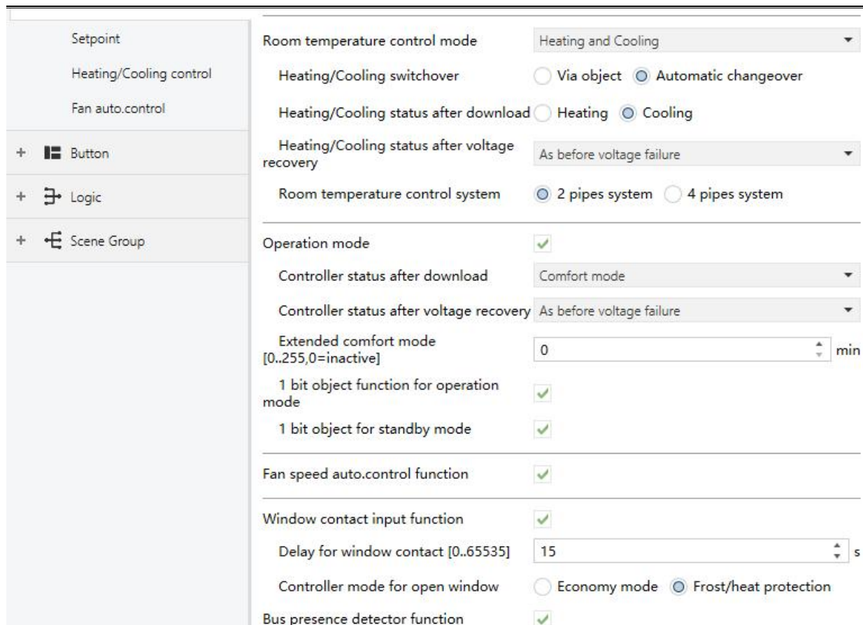
Fig.5.4.1 “Controller x - RTC” parameter window
