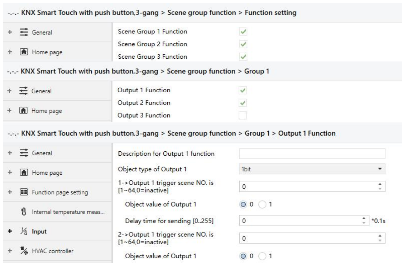
Fig.5.9 “Scene Group” parameter window
