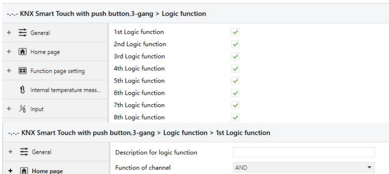
Fig.6.6 “Logic function setting” parameter window
