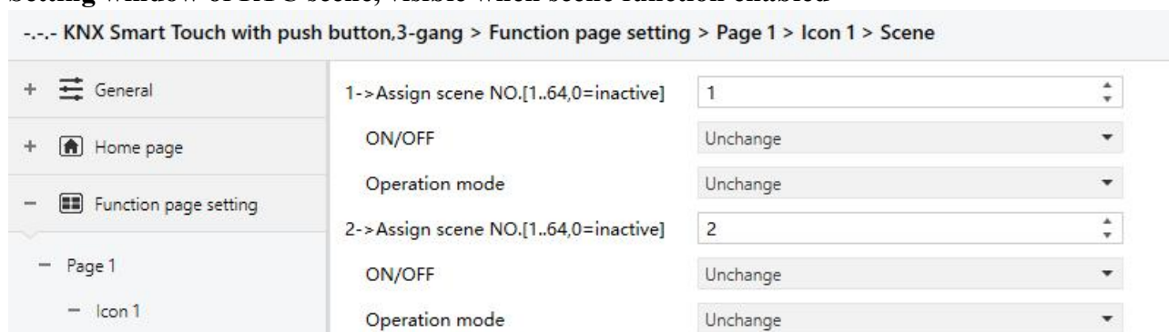
Fig.5.6.2.3(3) RTC -Scene parameter window
