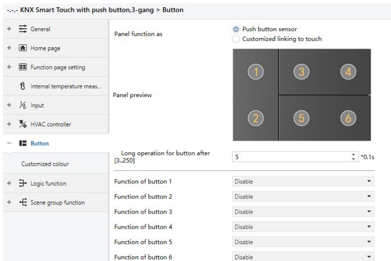
Fig.5.7.1 Parameter setting of button function
