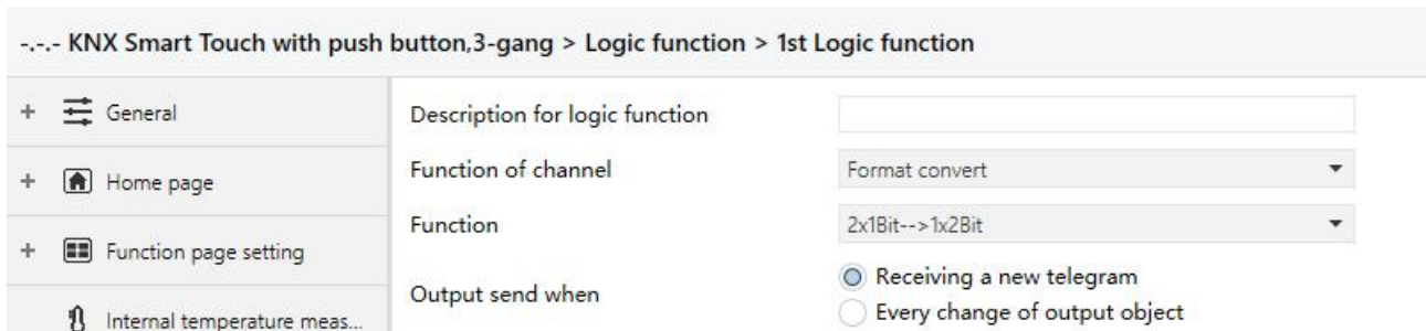
Fig.5.8.4 “Format convert” parameter window
