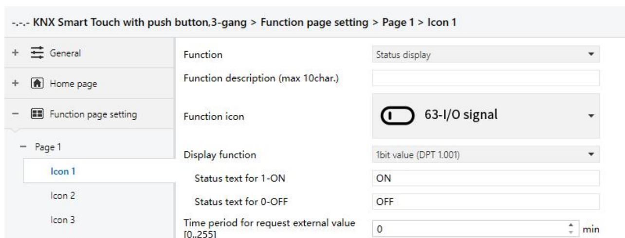
Fig.5.6.2.1(8) Parameter setting of status display
