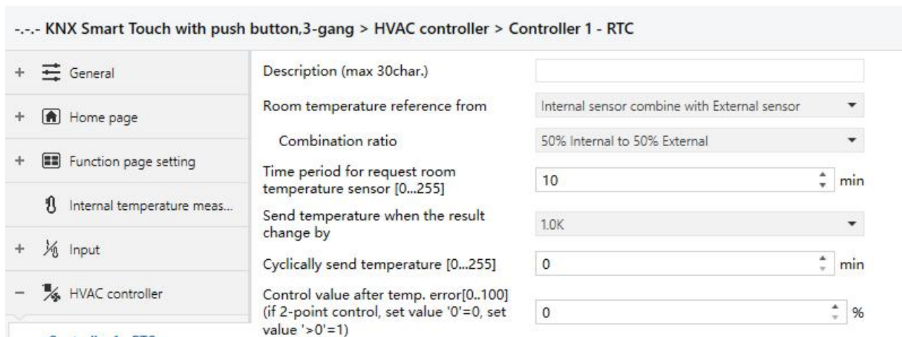
Fig.5.4.1 “Controller x - RTC” parameter window
