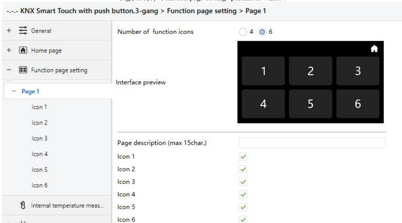
Fig.5.6.1(2) “Page x” parameter window
