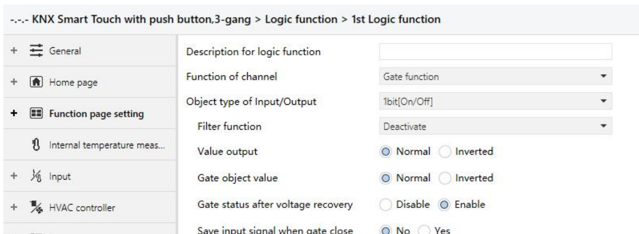
Fig.5.8.5 “Gate function” parameter window
