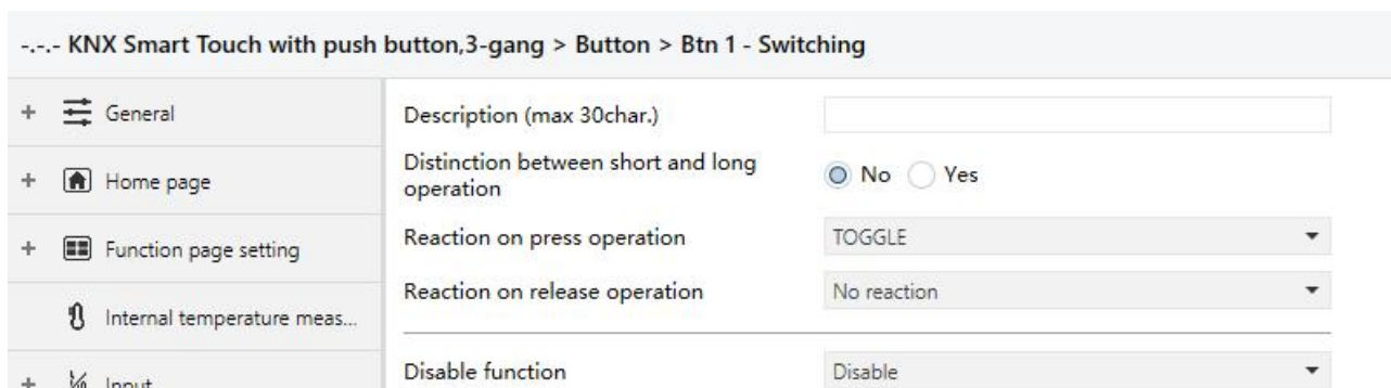
Fig.5.7.1.1 Parameter setting of switch function
