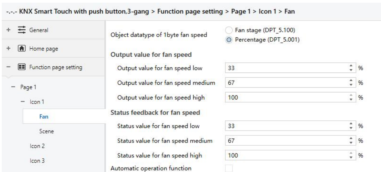
Fig.5.6.2.3(2) RTC -Fan speed parameter window
