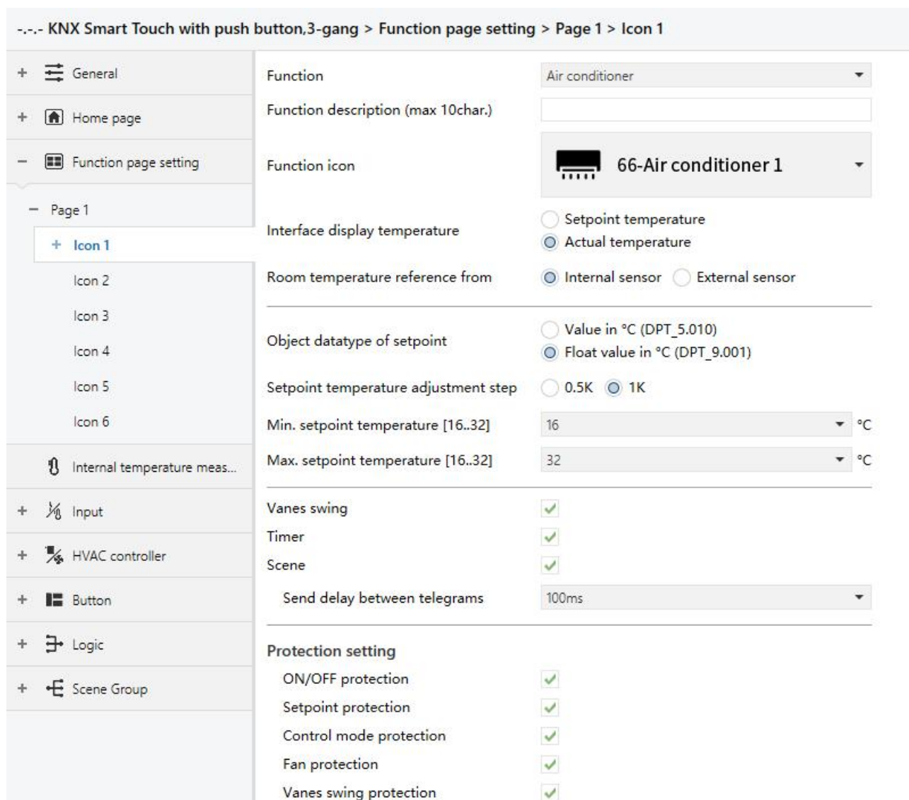
Fig.5.6.2.2(1) Air condition parameter window
